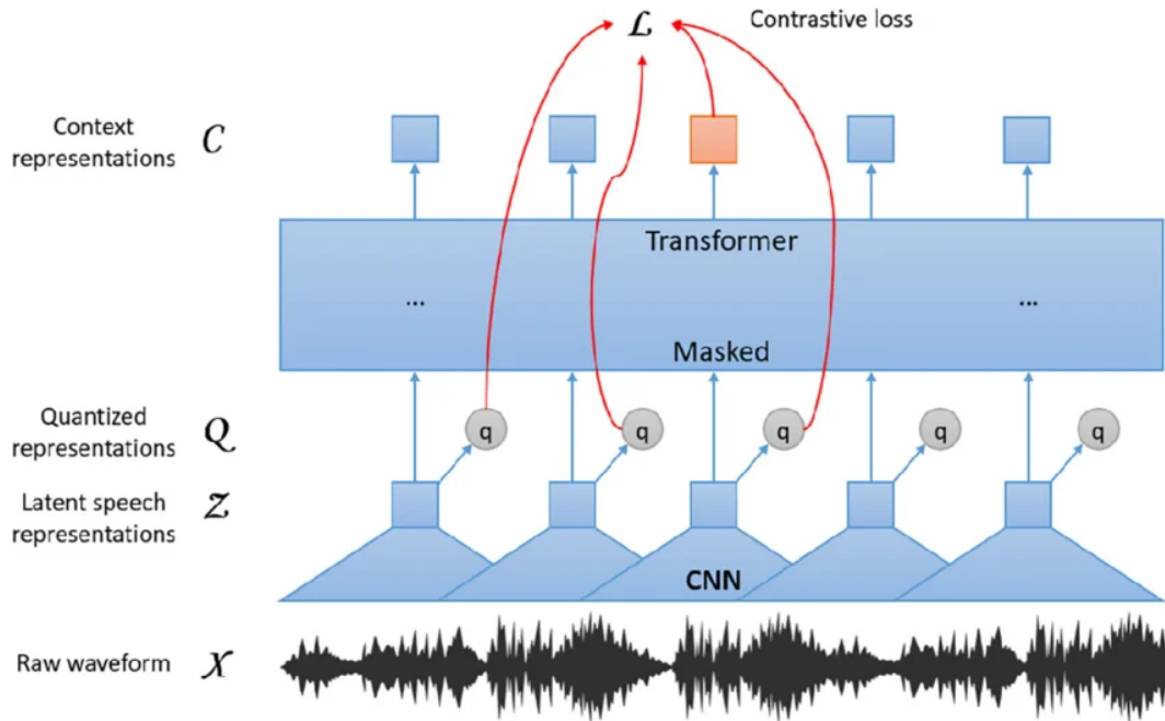
Gambar 2.5 Arsitektur Wav2Vec2 Sumber : Ovalle et al. (2024)
