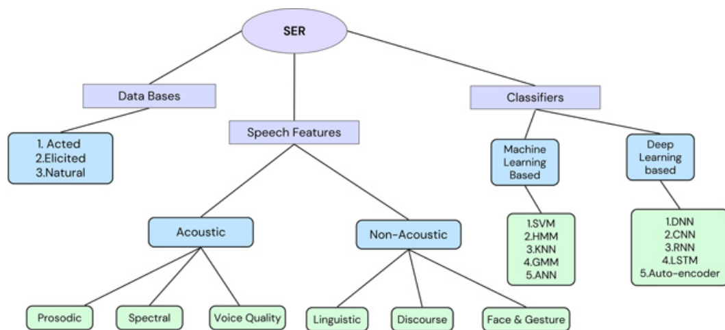
Gambar 2.1 Cakupan basis data, fitur, dan classifier pada SER
