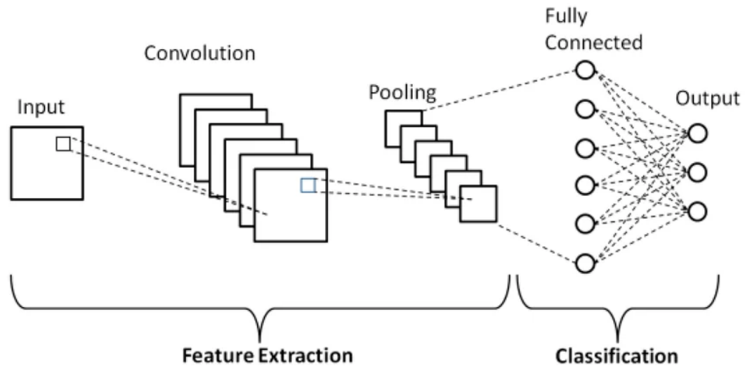
Gambar 2.3 Arsitektur umum Convolutional Neural Network (CNN)
